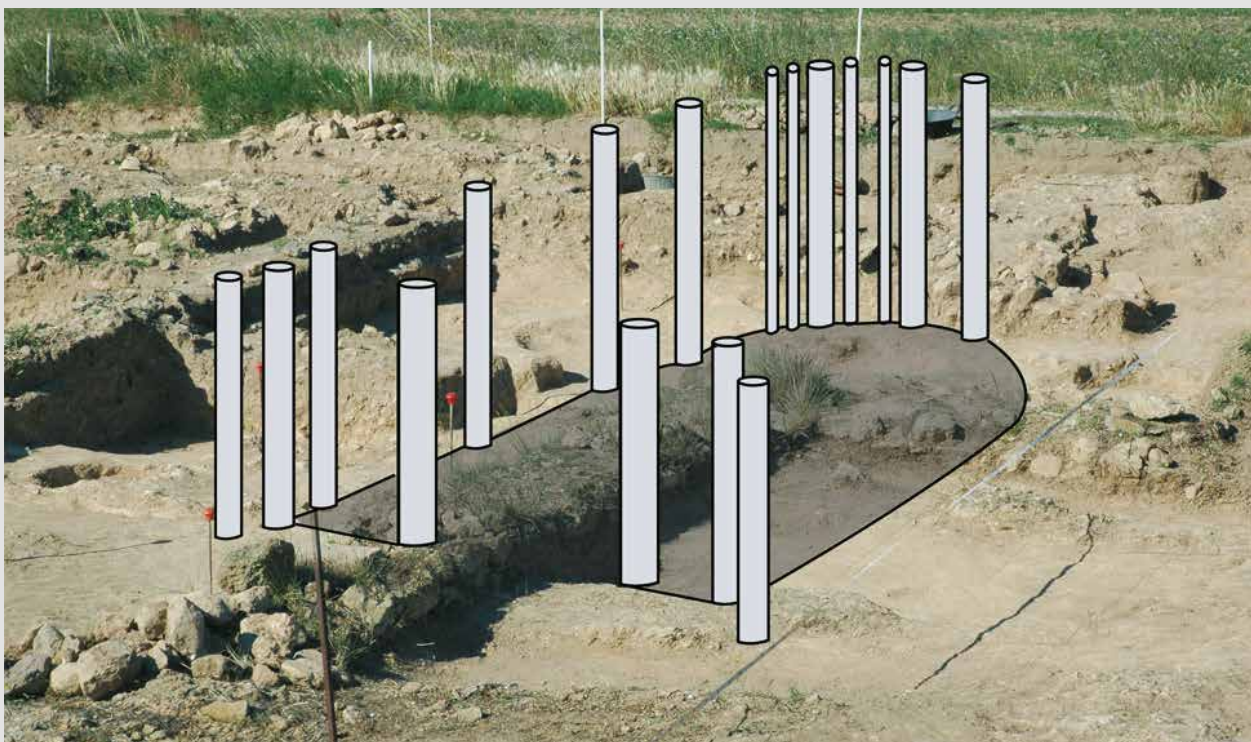
Casa de la primera edat del ferro a Mas Gusó (Bellcaire d'Empordà). Projecció vertical dels forats de pal identificats a l'excavació.
